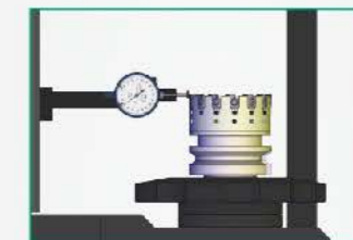
刀刃外徑校正
